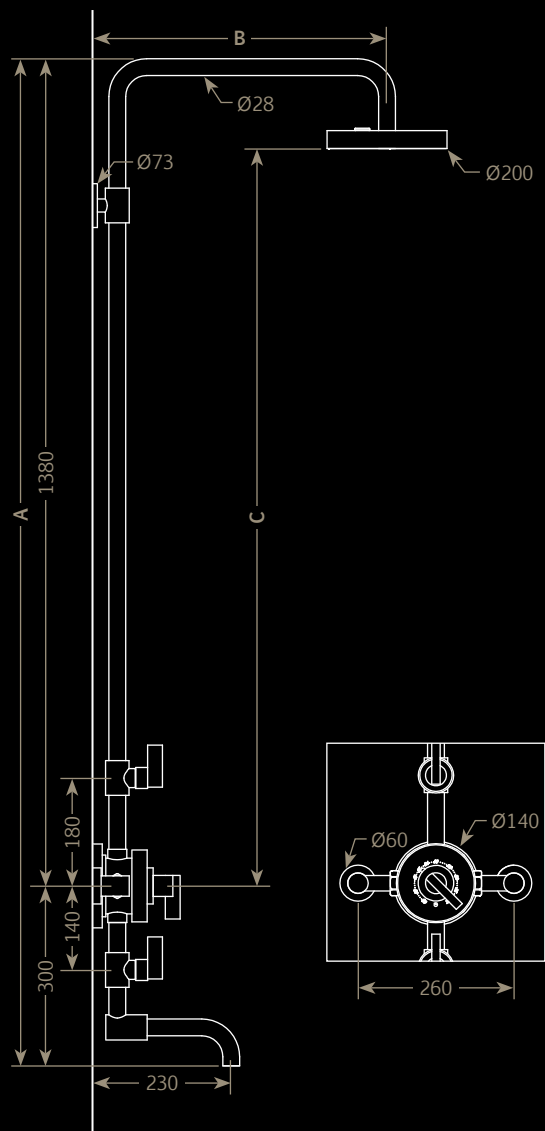
Ensemble externe avec mitigeur thermostatique, douche et bain Exposed shower system with thermostatic valve, shower head and tub spout
