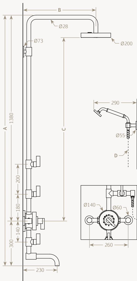
Ensemble externe avec mitigeur thermostatique, douche, douchette et bain Exposed shower system with thermostatic valve, shower head, handshower and tub spout
