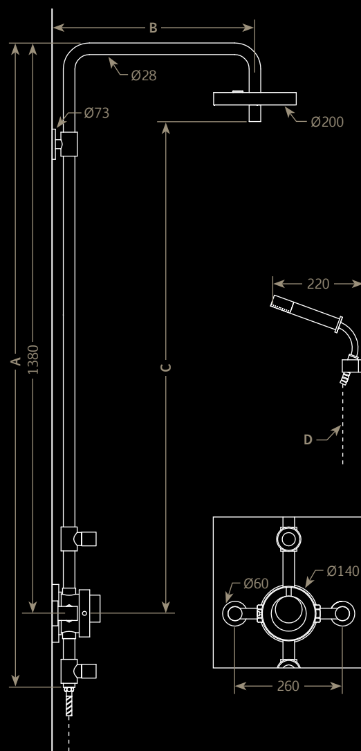
Ensemble externe avec mitigeur thermostatique, douche et douchette Exposed shower system with thermostatic valve, shower head and handshower
